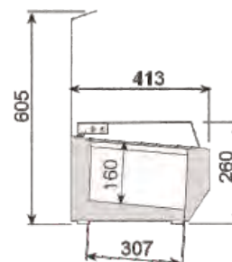
VIP 1/3 T TAPA / LID / COUVERCLE INOX
