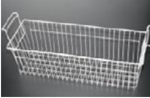
Cesto / Basket Dim. (mm): 765x275x230
